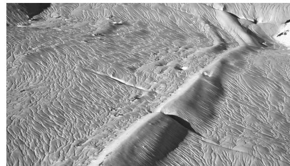
Seitenmoräne des Gruebengletschers. Foto: Mai 2004
